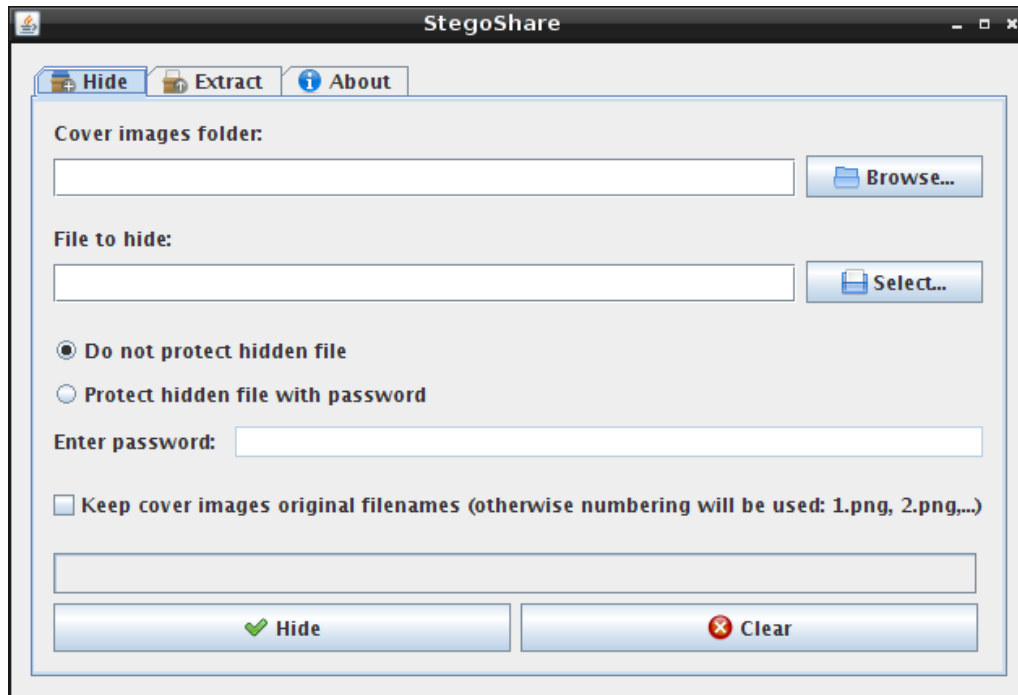
Рис. 4.10: Интерфейс StegoShare
