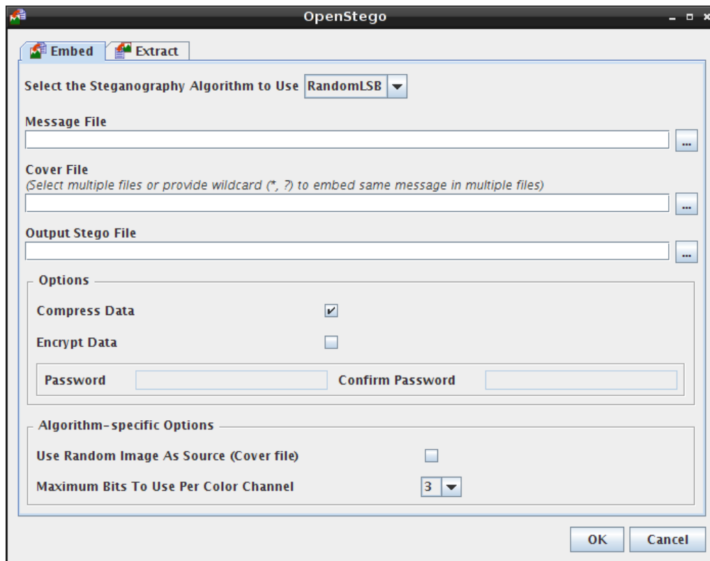
Рис. 4.8: Интерфейс OpenStego
